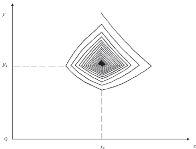
Рис. 4. Динамика правовой подсистемы в случае, когда макропеременная X оказывает антагонистическое влияние на Y , а макропеременная Y кооперативно действует на X (при s \ll \infty )
