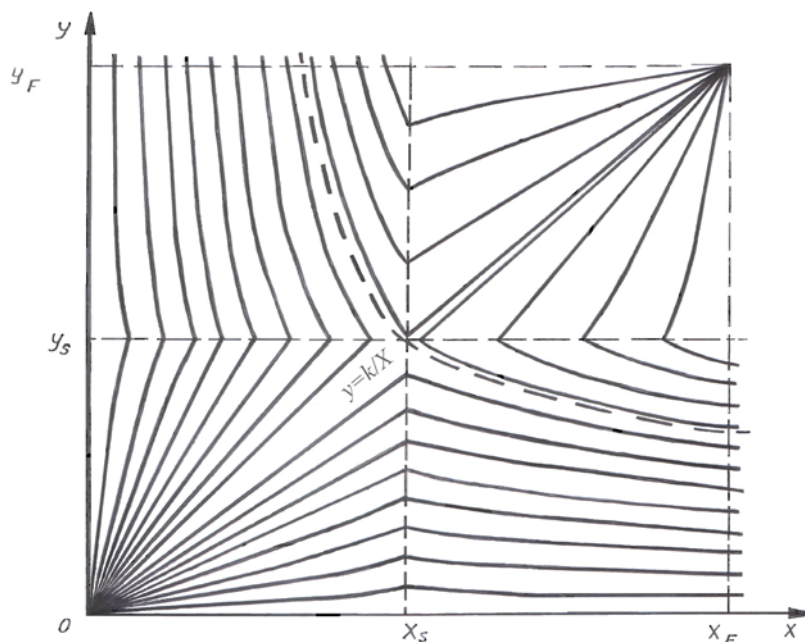
Рис. 2. Динамика правой подсистемы в случае кооперативного взаимовлияния макропеременных X и Y
